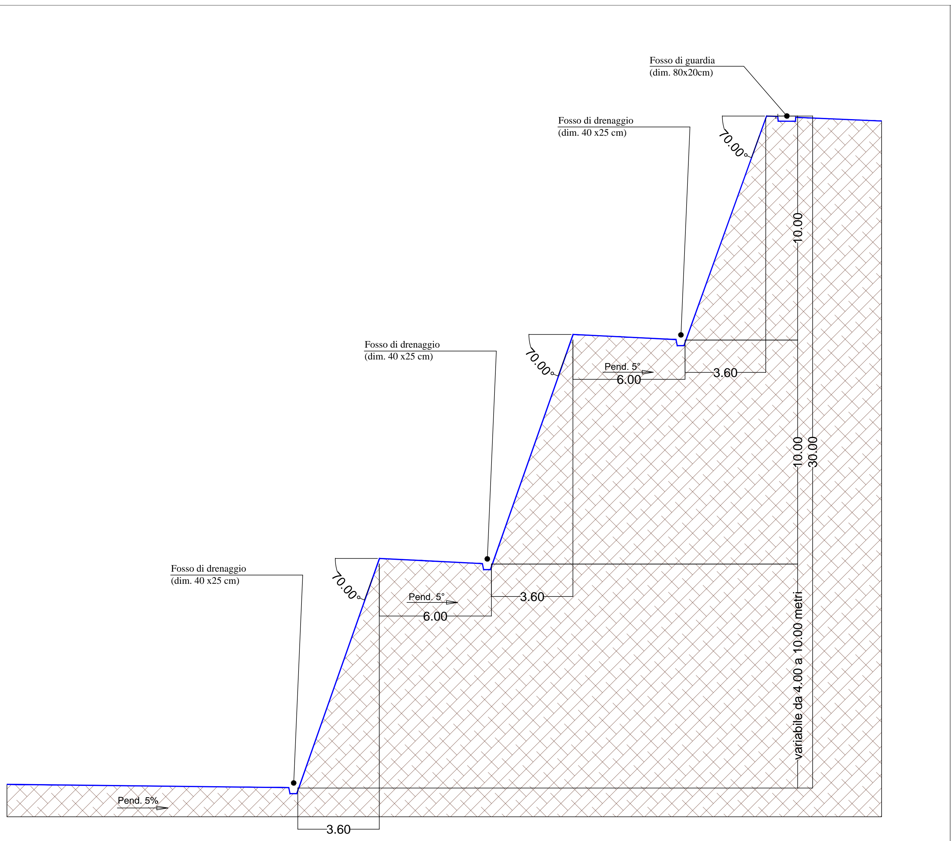
PARTICOLARE SEZIONE VERTICALE - SCAVO COMPLETO Rapporto di scala 1:100
