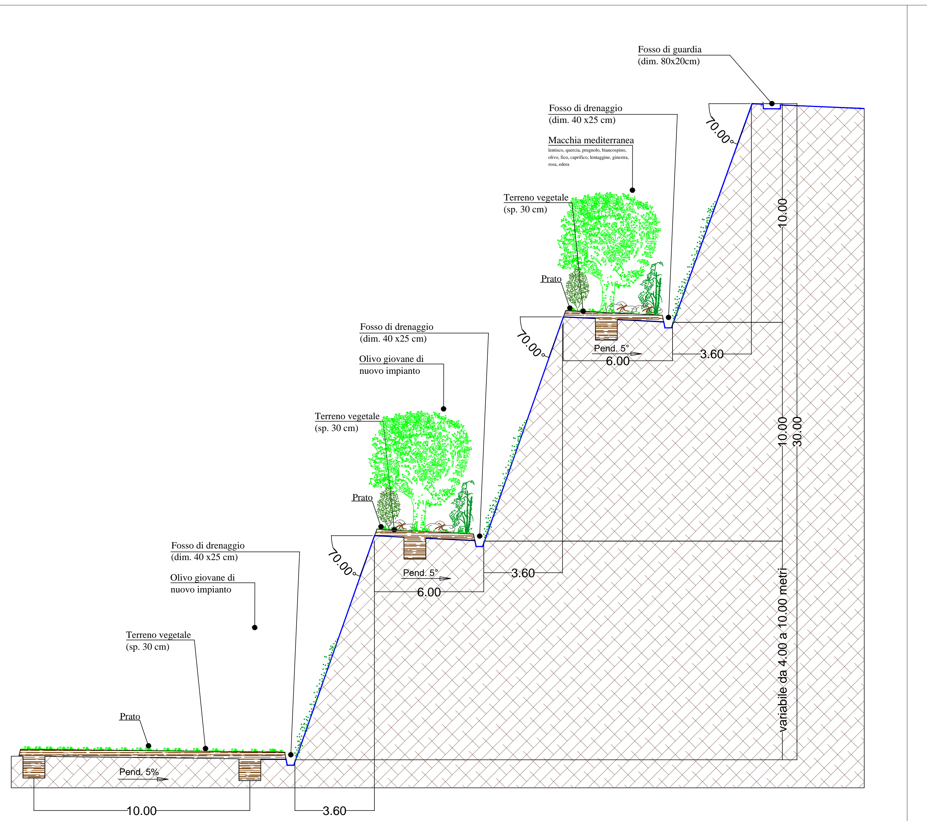
PARTICOLARE SEZIONE VERTICALE - RECUPERO AMBIENTALE 1 Rapporto di scala 1:100
