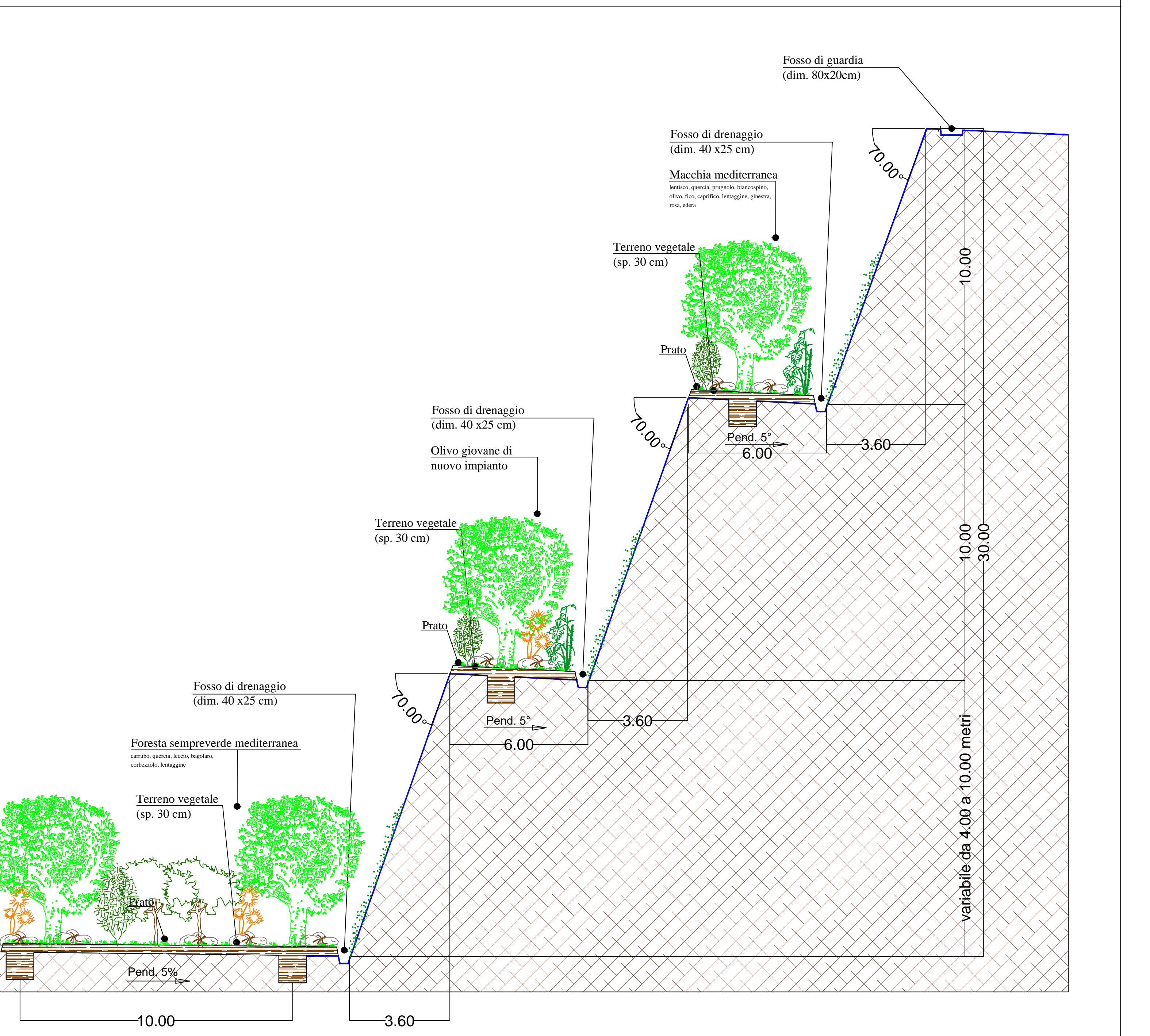
PARTICOLARE SEZIONE VERTICALE - RECUPERO AMBIENTALE 2 Rapporto di scala 1:100
