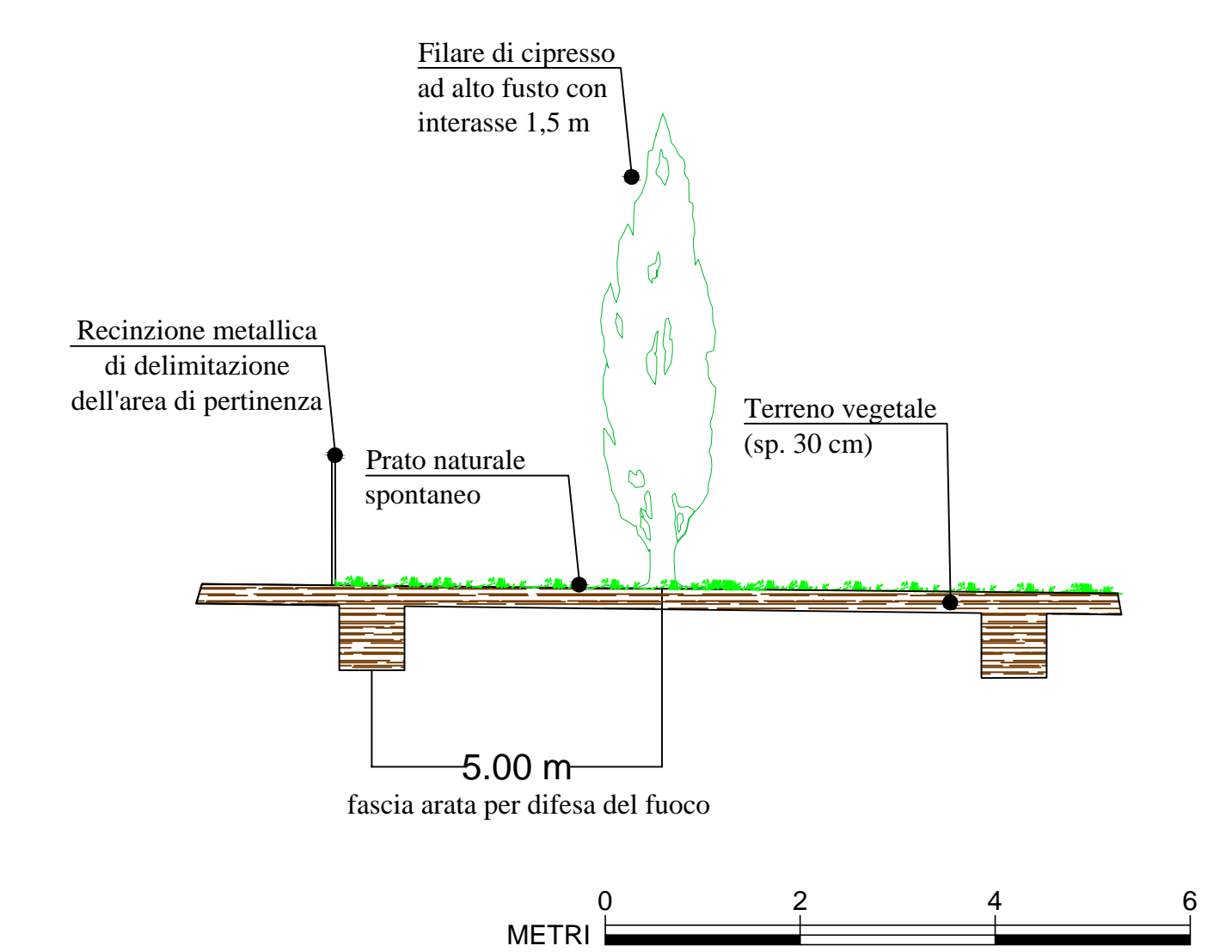
PARTICOLARE SEZIONE VERTICALE RECINZIONE AREA DI PERTINENZA Rapporto di scala 1:100
